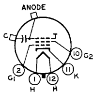
12N Anode = G_2 + CL
