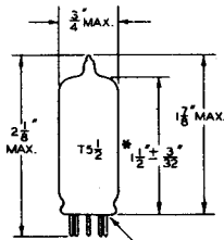
5-2 Bouton miniature 7 broches
