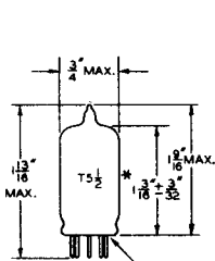
5-1 Bouton miniature 7 broches
