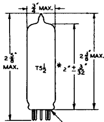
5-3 Bouton miniature 7 broches
