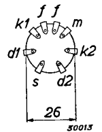
Abb. 2 Elektrodenanordnung und Sockelanschlüsse.
